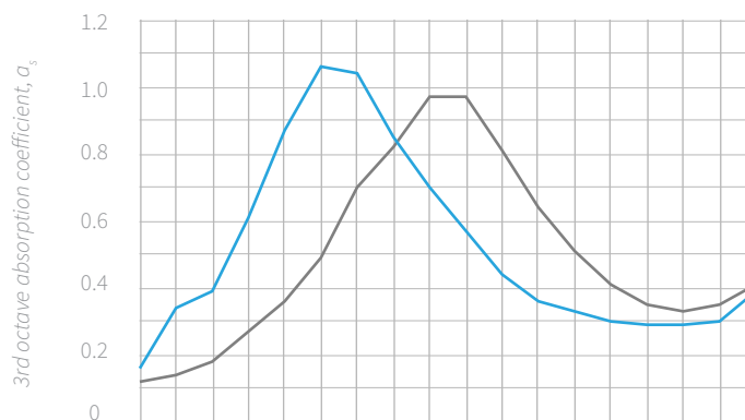
Absorption data for Groove 24 (EN 354: 2003)
