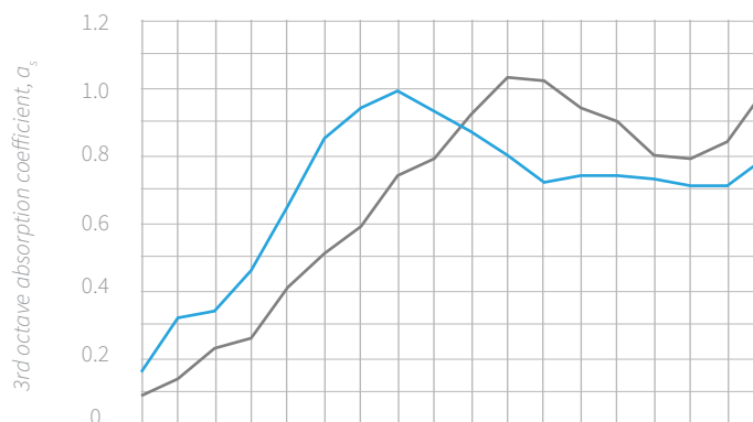
Absorption data for Groove 5-H (EN 354: 2003)
